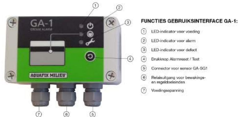
Afbeelding 2. Functies van regeleenheid GA-1
