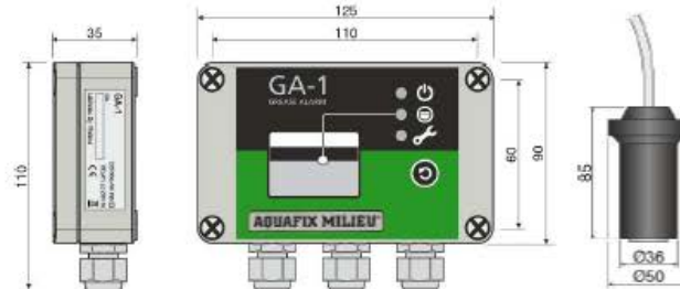
Afbeelding 7. Regeleenheid GA-1
